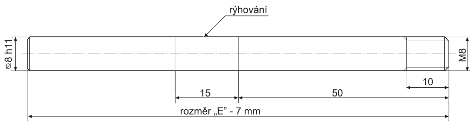
Obr. 31: Náskres měřicí elektrody s vyznačeným závitem pro připojení a rýhováním
