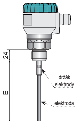
Obr. 30: Nákres hladinoměru s rozměrem "E"
