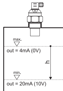
Fig. 32: Inverse mode
