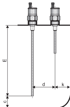
Obr. 1: Svislá instalace snímačů
