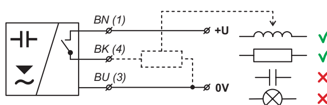
Obr. 2: zapojení snímače s výstupem typu „P“ (PNP)
