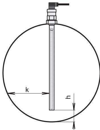
Obr. 5: Instalace hladinoměru s referenční trubkou
