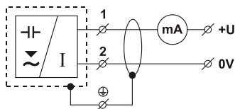
Obr. 9: Připojovací schéma hladinoměru s proudovým výstupem
