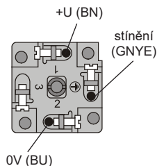
Obr. 10: Vnitřní pohled na konektor s proudovým výstupem
