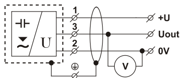
Obr. 11: Připojovací schéma hladinoměru s napětovým výstupem
