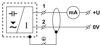
Obr. 6: Připojovací schéma hladinoměru s proudovým výstupem
