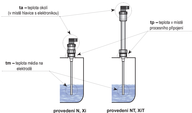
Obr. 14: Body pro stanovení teplot na hladinoměru
