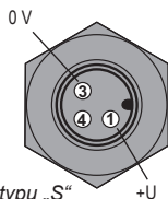
Obr. 22: Schéma připojení snímače ULS s výstupem typu „S“ (dvoustavový proudový spínač 4,41A / 20 mA)
