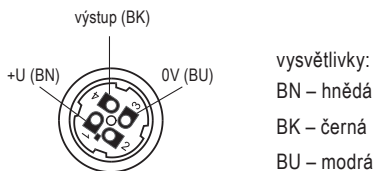
Obr. 19: Vnitřní pohled na konektorovou zásuvku
