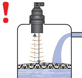
Obr. 5: Pěna na hladině
