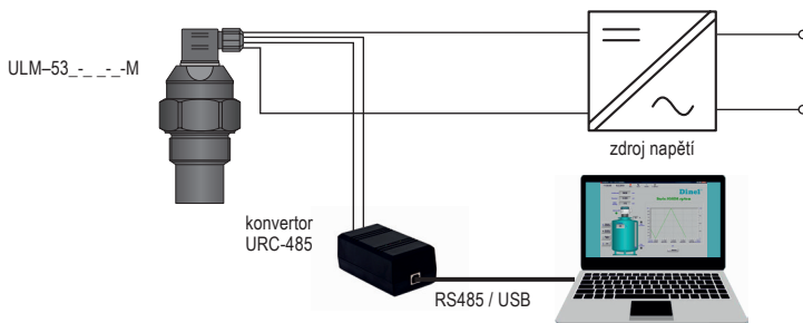
Obr. 23: Připojení periferních zařízení protokolem Modbus®
