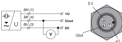
Obr. 21: Schéma připojení hladinoměru ULM (varianta -U) a pohled na konektor
