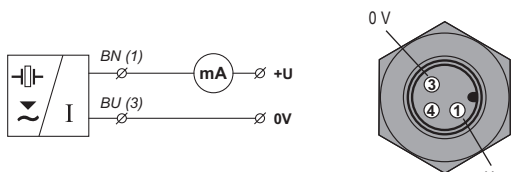
Obr. 20: Schéma připojení hladinoměru ULM (varianta -I) a pohled na konektor
