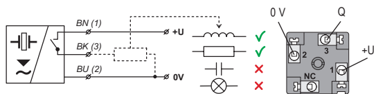
Obr. 18: Schéma připojení snímače ULS s výstupem typu „P“ (PNP) s otevřeným kolektorem
