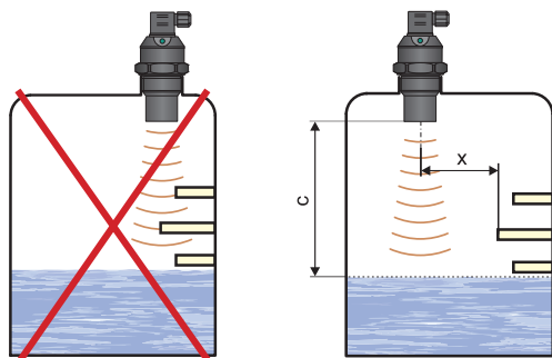
Obr. 6: Minimální vzdálenost hladinoměru od blízkých předmětů v nádrži
