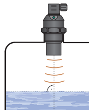
Obr. 1: Správná instalace hladinoměru kolmo na hladinu kapaliny
