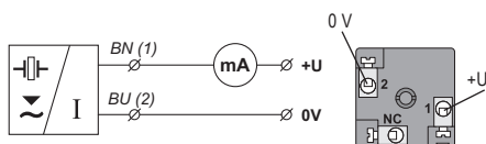
Obr. 15: Schéma připojení hladinoměru ULM (varianta –I) a vnitřní pohled na konektor
