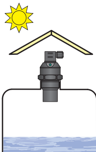
Obr. 8: Stínící kryt proti přímému slunečnímu záření
