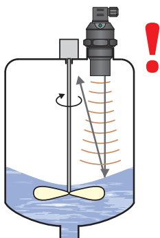
Obr. 11: Silně rozvířená hladina
