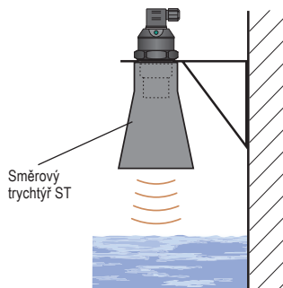
Obr. 13: Instalace směrového trychtýře
