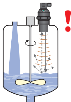
Obr. 10: Mírně zvlněná hladina
