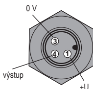
Obr. 23: Schéma připojení snímače ULS s výstupem typu „P“ (PNP) s otevřeným kolektorem
