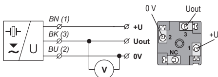
Obr. 16: Schéma připojení hladinoměru ULM (varianta –U) a vnitřní pohled na konektor
