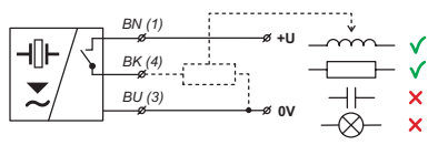
Obr. 23: Schéma připojení snímače ULS s výstupem typu „P“ (PNP) s otevřeným kolektorem
