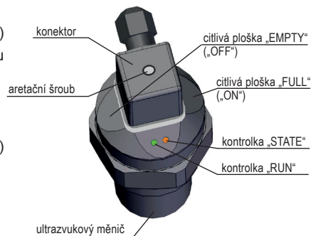
Obr. 30: Hlavní části měřícího zařízení (verze s hallovými sondami)
