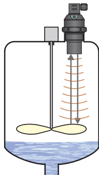
Obr. 12: Falešný odraz od lopatek míchadla
