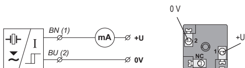
Obr. 17: Schéma připojení snímače ULS s výstupem typu „S“ (dvoustavový proudový spínač 4 mA / 20 mA)
