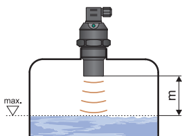
Obr. 2: Mrtvá zóna hladinoměru
