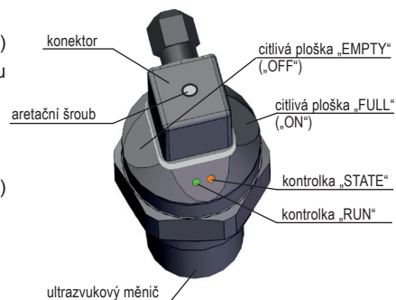
Obr. 30: Hlavní části měřícího zařízení (verze s hallovými sondami)
