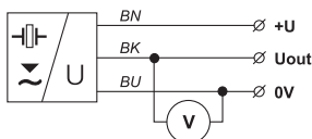
Obr. 25: Schéma připojení hladinoměru ULM s napěťovým výstupem (varianta -U)
