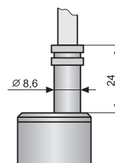
Provedení "B" dlouhá kabelová vývodka
