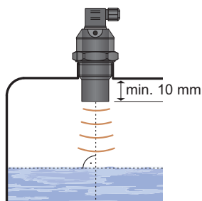
Doporučená instalace hladinoměru ULS-53 v nádrži
