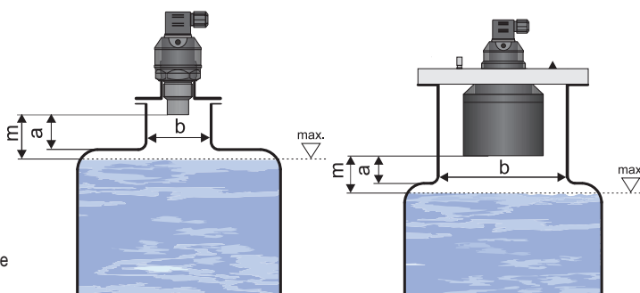
Instalace hladinoměř ULS-53 přes vstupní hrdlo (tímto způsobem je možné nádrž zaplnit téměř do maximální výšky)
