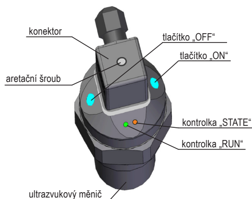
Popis hlavních částí snímače verze "T" s tlačítky
