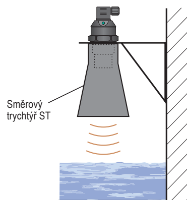
Instalace směrového trychtýře
