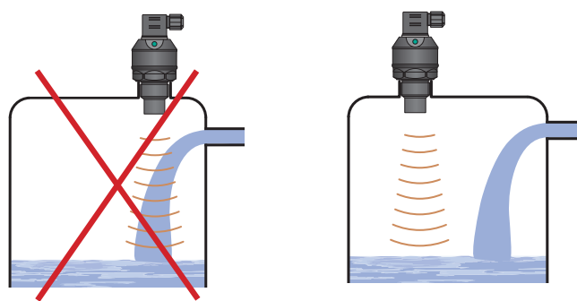
Instalace zařízení mimo dosah plnicího proudění
