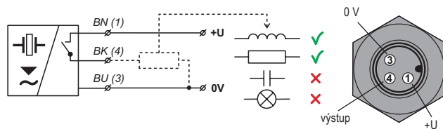
Připojovací schéma a vnitřní pohled na konektor snímače ULS s výstupem typu „P“ (PNP) s otevřeným kolektorem
