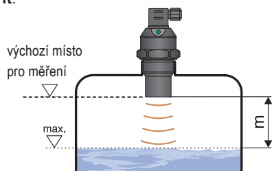
Mrtvá zóna hladinoměů
