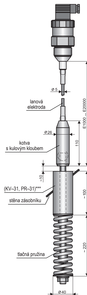
CLM - 36_-31
