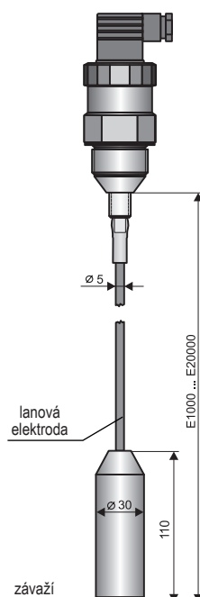
CLM - 36_-30
