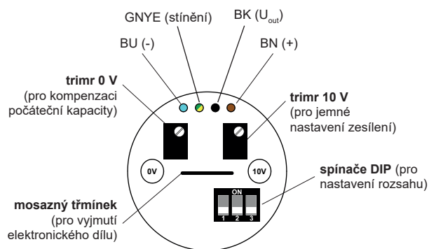
pohled shora na vnitřní elektronický díl hladinoměru s napěťovým výstupem (varianta –U)
