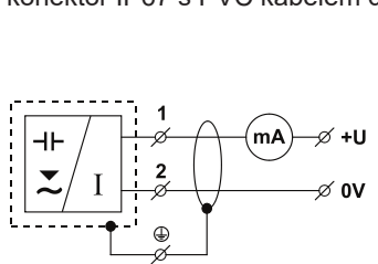
Připojovací schéma hladinoměru s proudovým výstupem
