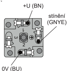
Vnitřní pohled na konektor s proudovým výstupem
