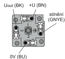
Vnitřní pohled na konektor s napěťovým výstupem
