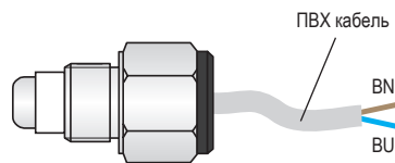
Рис. 1: Подключение кабеля у варианта CNP-18N
