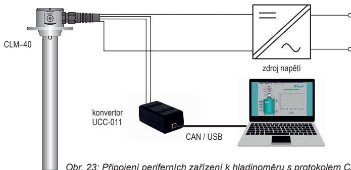
Obr. 23: Připojení periferních zařízení k hladinoměru s protokolem CAN
