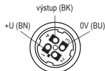
Obr. 16: Vnitřní pohled na konektorovou zásuvku
