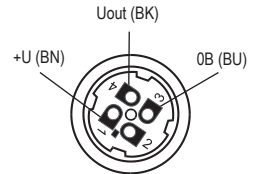
Рис. 6: Вид изнутри гнезда разъёма (вариант "C")
