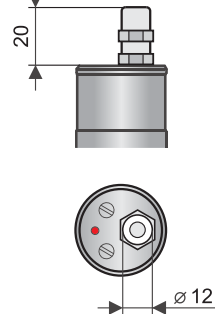
provedení "D" s kab. vývodkou
