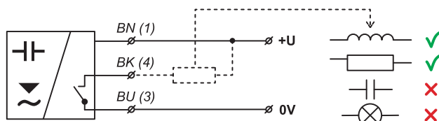
zapojení snímače s výstupem typu NPN (provedení N; NT; Xd)
