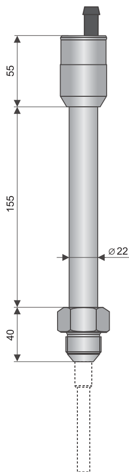
vysokoteplotní provedení
