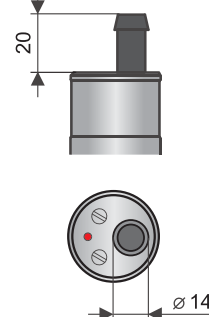
provedení "B" s kab. vývodkou
