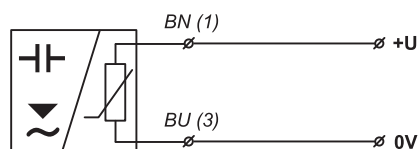
zapojení snímače s výstupem typu NAMUR (provedení Xi; XiT; XiM; XiMT)
