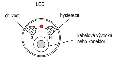
pohled shora na snímač
