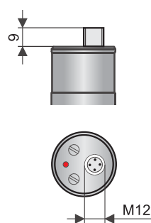
provedení "C" s konektorem
