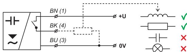
zapojení snímače s výstupem typu PNP (provedení N; NT; Xd)
