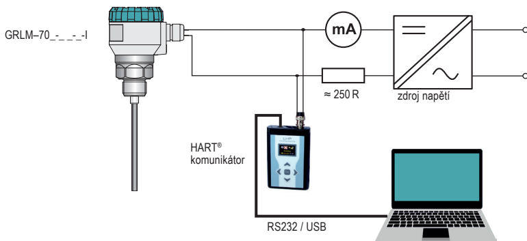
Obr. 25: Připojení periferních zařízení s protokolem HART
