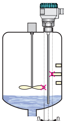
Obr. 13: Nesprávná instalace hladinoměru v blízkosti překážek
