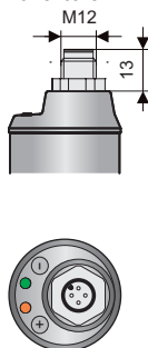
Provedení "C" s konektorem M12
