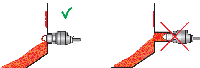
Obr. 3: Správná a nevhodná instalace s dlouhým nátrubkem
