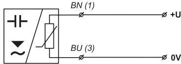
Obr. 7: Zapojení snímače s výstupem typu NAMUR (provedení Xi a XiM)
