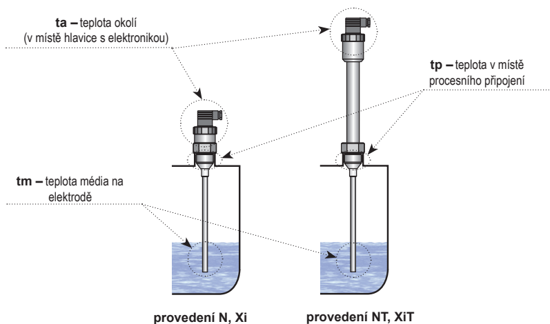
Obr. 14: Body pro stanovení teplot na hladinoměru
