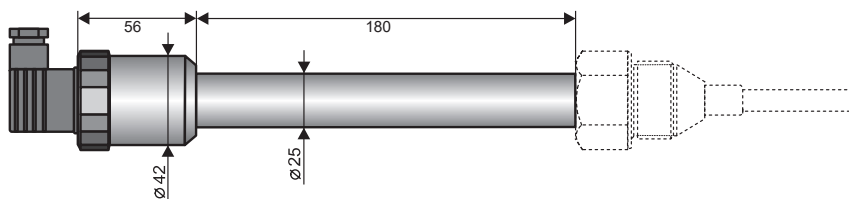
vysokoteplotní provedení CLM-36_T
