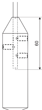
Obr. 13: Náčrtes závaží lanové elektrody
