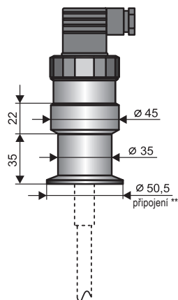
Procesní připojení Tri-clamp
