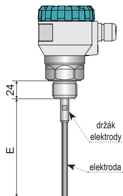
Obr. 27: Nákres hladinoměru s rozměrem "E"
