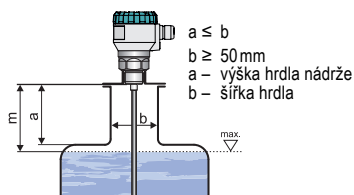
Obr. 5: Instalace hladinoměru ve vstupním hrdle
