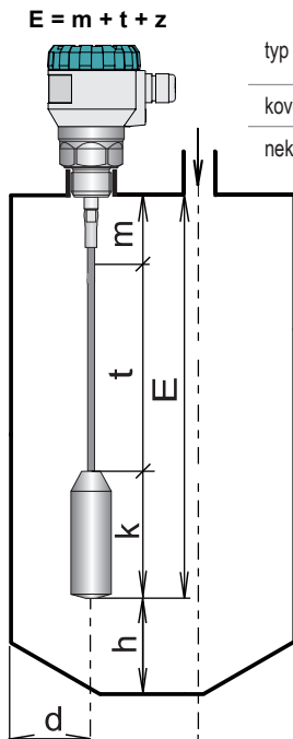
Obr. 2: Instalace hladinoměru s lanovou elektrodou
