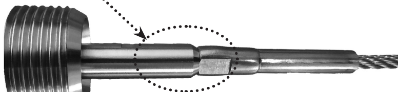
Obr. 30 Zobrazení závitového spoje držáku elektrody s lanovou elektrodou
