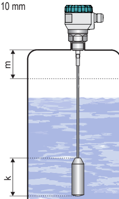
Obr. 4: Mrtvé zóny hladinoměru s lanovou elektrodou
