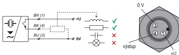
Obr. 25: Schéma připojení snímače ULS s výstupem typu „P“ (PNP) s otevřeným kolektorem
