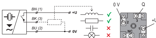
Obr. 20: Schéma připojení snímače ULS s výstupem typu „P“ (PNP) s otevřeným kolektorem
