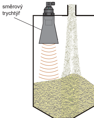
Obr. 14: Instalace hladinoměru v síle nebo zásobníku
