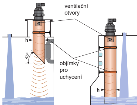
Obr. 6: Použití zkrácené vodící trubky
