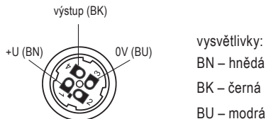
Obr. 21: Vnitřní pohled na konektorovou zásuvku
