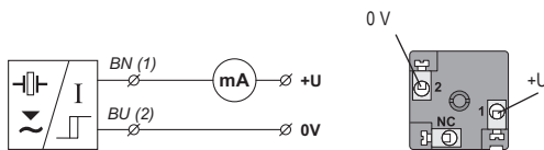
Obr. 19: Schéma připojení snímače ULS s výstupem typu „S“ (dvoustavový proudový spínač 4 mA / 20 mA)
