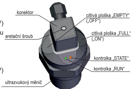
Obr. 32: Hlavní částí měřicího zařízení (verze s hallovými sondami)
