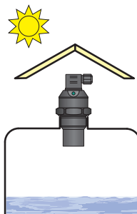
Obr. 15: Stínící kryt proti přímému slunečnímu záření
