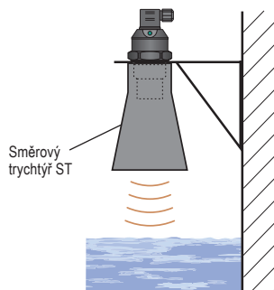
Obr. 8: Instalace směrového trychtýře
