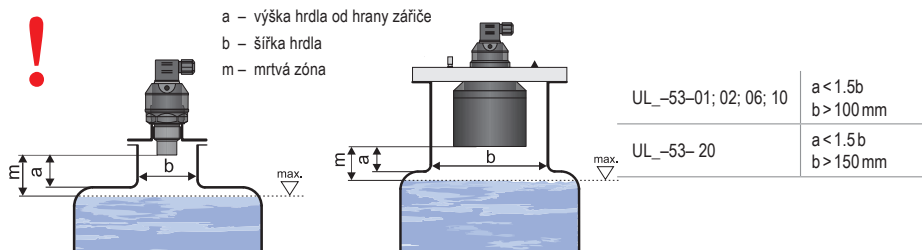
Obr. 5: Instalace hladinoměru ve vstupním hrdle
