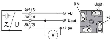
Obr. 18: Schéma připojení hladinoměru ULM (varianta –U) a vnitřní pohled na konektor
