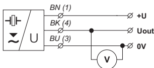
Obr. 23: Schéma připojení hladinoměru ULM (varianta -U) a pohled na konektor
