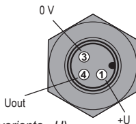
Obr. 23: Schéma připojení hladinoměru ULM (varianta -U) a pohled na konektor
