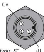
Obr. 24: Schéma připojení snímače ULS s výstupem typu „S“ (dvoustavový proudový spínač 4 mA / 20 mA)
