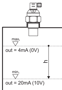
Obr. 34: Inverzní režim
