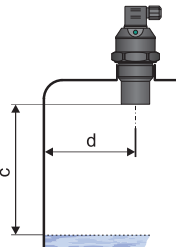
Obr. 3: Vzdálenost hladinoměru od stěny nádrže
