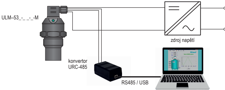
Obr. 35: Připojení periferních zařízení protokolem Modbus®
