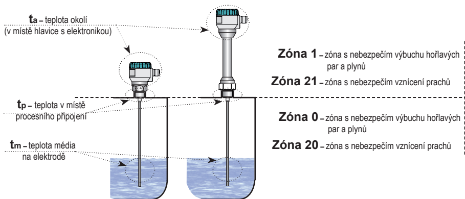
Obr. 34: Zobrazení oblastí pro měření teplot a zón výbušnosti
