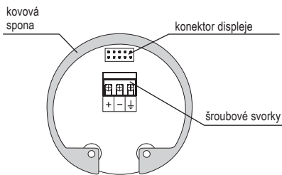
Obr. 20: Vnitřní pohled na šroubové svorky hladinoměru s proudovým výstupem GRLM-70_--_-I
