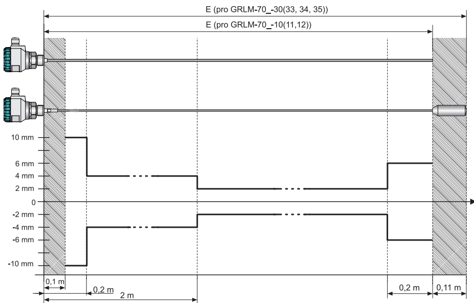
Obr. 33 Graf závislosti chyby měření podél tyčové a lanové elektrody
