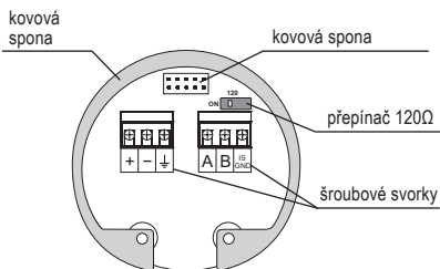
Obr. 22: Vnitřní pohled na šroubové svorky hladinoměru s komunikací Modbus GRLM-70_--_-M
