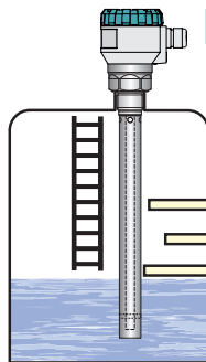
Obr. 14: Instalace hladinoměru s referenční trubicou do stísněných prostorů
