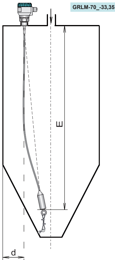
Obr. 17: Doporučená instalace hladinoměru s kotvením
