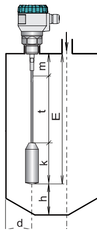
Obr. 16: Instalace hladinoměru s lanovou elektrodou
