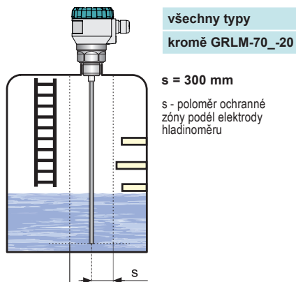
Obr. 12: Instalace hladinoměru mimo překážky v nádrži
