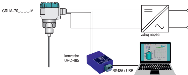
Obr. 26: Připojení periferních zařízení protokolem Modbus®
