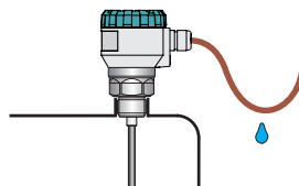
Obr. 15: Zamezení proti vniknutí vlhkosti kabelovou průchodkou
