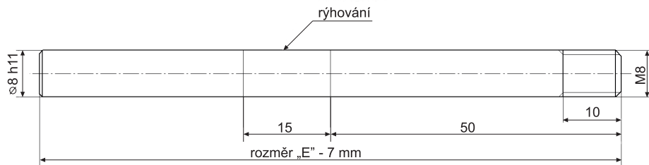
Obr. 28: Nákres měřicí elektrody s vyznačeným závitem pro připojení a rýhováním
