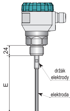
Obr. 27: Nákres hladinoměru s rozměrem "E"
