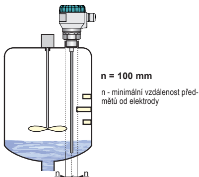
Obr. 24: Nasměrování lopatky míchadla do blízkosti elektrody před spuštěním režimu "Učení"
