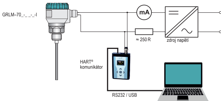
Obr. 25: Připojení periferních zařízení s protokolem HART
