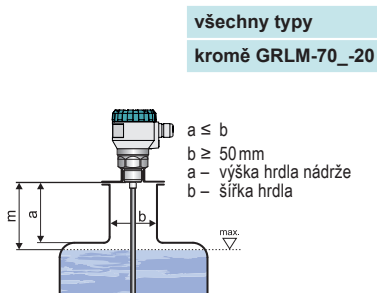
Obr. 5: Instalace hladinoměru ve vstupním hrdle
