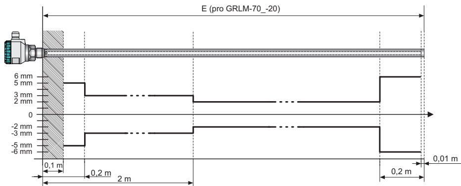
Obr. 32: Graf závislosti chyby měření podél tyčové elektrody s referenční trubicou
