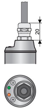
Provedení "D" s kovovou prachotěsnou vývodkou
