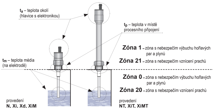
Obr. 15: Zobrazení oblastí pro měření teplot a zón výbušnosti
