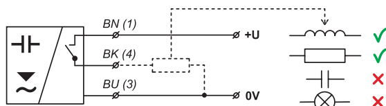
Obr. 14: Zapojení snímače s výstupem typu PNP (provedení N, NT, Xd)
