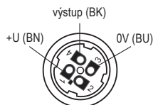
Obr. 16: Vnitřní pohled na konektorovou zásuvku
