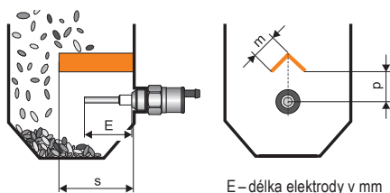
Obr. 4: Montáž ochranné stříšky
