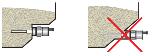
Obr. 5: Montáž do šikmé stěny zásobníku
