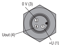
Obr. 8: Připojení konektoru na snímači
