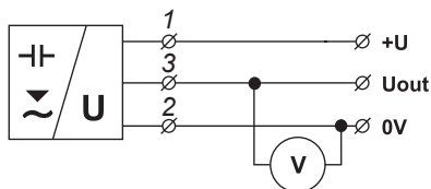
Připojení hladinoměru s napěťovým výstupem
