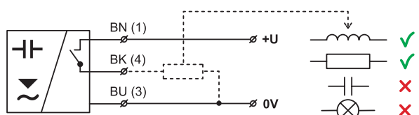
Подключение датчика с выходом типа PNP (вариант «P»)
