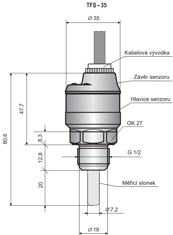
Provedení "B" s plastovou závitovou vývodkou
