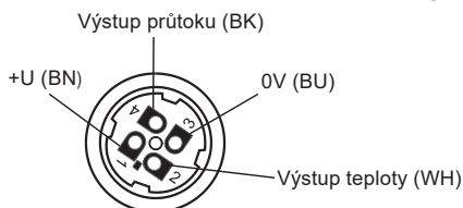
Vnitřní pohled na konektorovou zásuvku (varianta "C")
