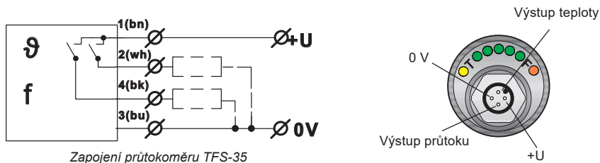
Zapojení průtokoměru TFS-35
