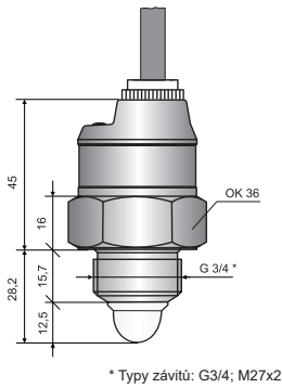
RFLS-35_-2-G3/4
