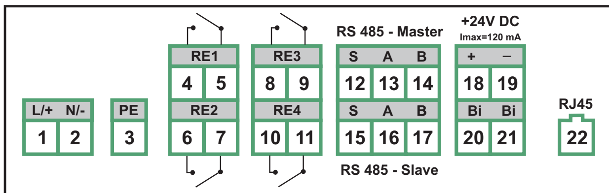
SVORKOVNICE FCU-400-R_-0(W)
