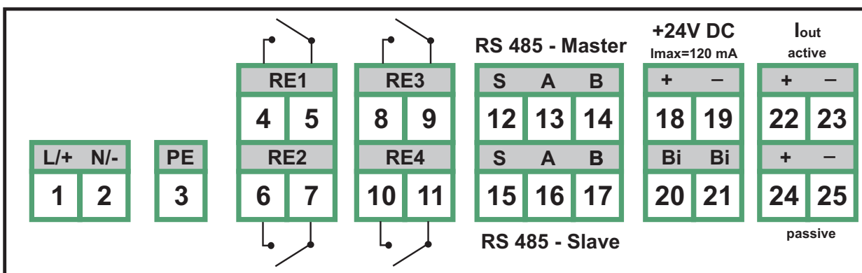
SVORKOVNICE FCU-400-R_-I
