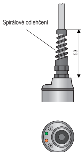
Provedení „V“ s plastovou vývodkou se spirálovým odlehčením - pro případ zvýšeného mechanického namáhání kabelu.
