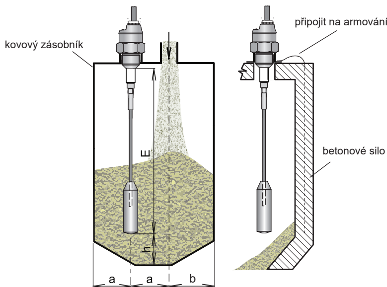
Instalace hladinoměru s lanovou elektrodou
