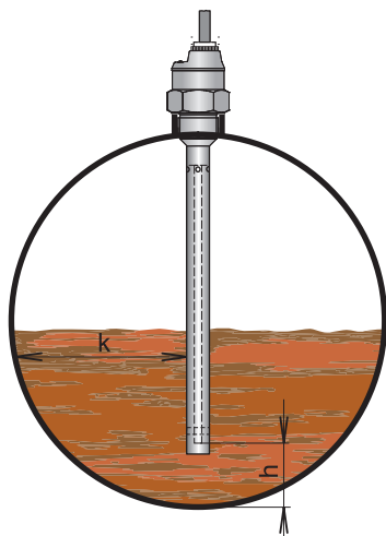
Instalace hladinoměru s referenční trubicou
