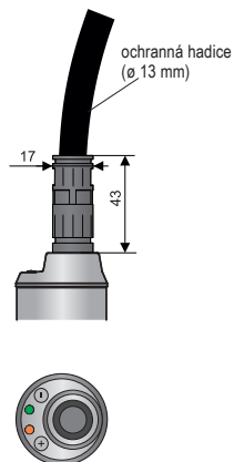
Provedení „H“ s vývodkou pro ochranné hadice - pro použití ve venkovním prostředí nebo v místě zvýšené vlhkosti.
