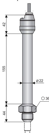
Provedení „C“ s konektorem M12
