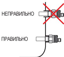
Рис. 5: Установка около впускных отверстий
