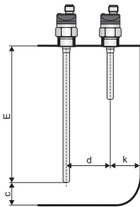
Рис. 1: Вертикальная установка датчиков
