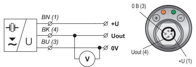
Схема подключения и вид изнутри разъёма уровнемера DLM (вариант - U)
