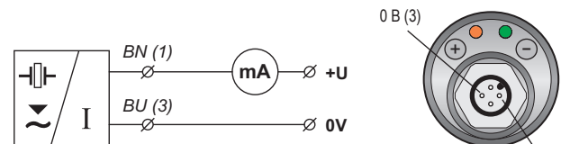
Схема подключения и вид изнутри разъёма уровнемера DLM (вариант - I)
