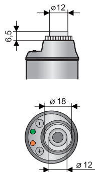
Provedení „A“ s krátkou nerez. vývodkou
