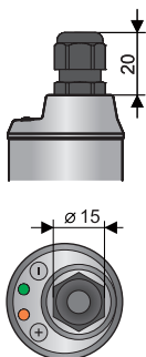
Provedení "B" se závitovou vývodkou
