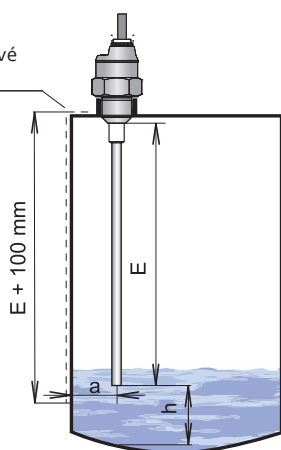
Obr. 19: Instalace hladinoměru s tyčovou elektrodou
