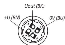
Obr. 24: Vnitřní pohled na konektorovou zásuvku (varianta "C")
