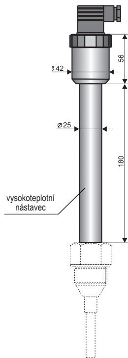
vysokoteplotní provedení CLM-36_T
