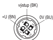
Vnitřní pohled na konektorovou zásuvku
