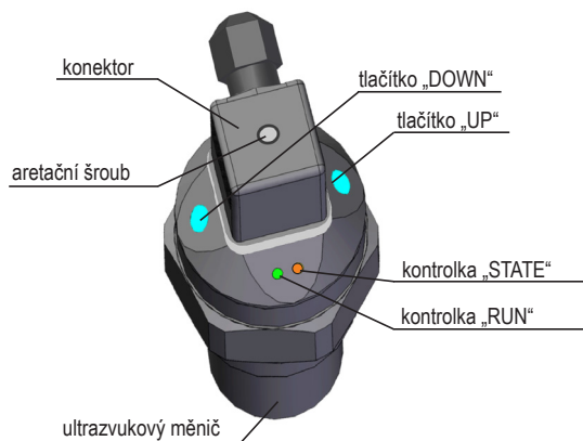
Popis hlavních částí snímače verze "T" s tlačítky
