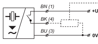
Schéma připojení snímače ULS s výstupem typu „P“ (PNP) s otevřeným kolektorem
