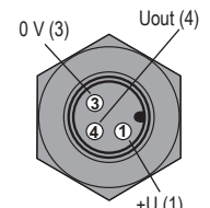
Schéma připojení snímače ULS s výstupem typu „P“ (PNP) s otevřeným kolektorem
