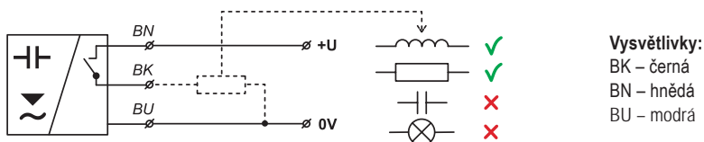
Obr. 1: Zapojení snímače RFLS-28_-_-P-_- s výstupem typu PNP
