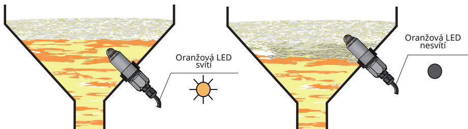
Obr. 11: Hlídání hladiny pěnivého média
