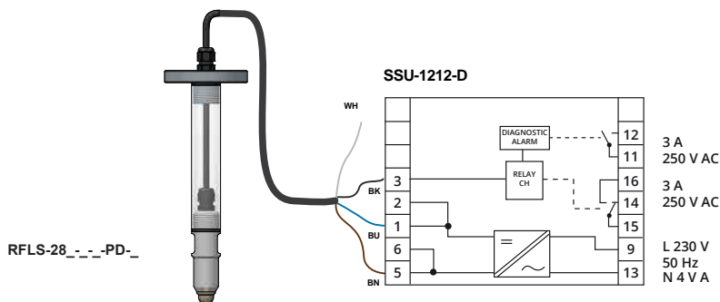
Obr. 3: Zapojení snímače do jednotky SSU-1212-D
