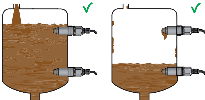
Obr. 8: Boční instalace snímačů do nádoby s viskózním médiem
