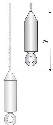
Obr. 29: Náčres zakončení lana pro typ 33, 35
