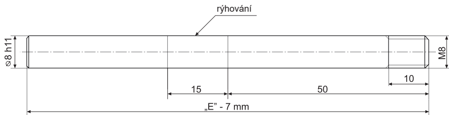
Obr. 24: Detail náčrtu tyčové elektrody
