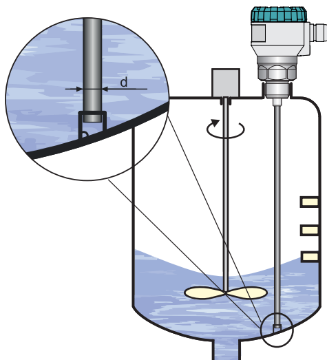
Obr. 23: Doporučená instalace hladinoměru s kotvením tyčové elektrody
