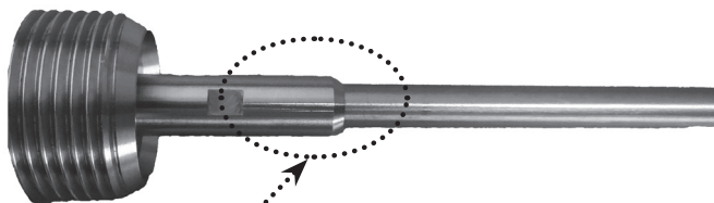
Obr. 26: Zobrazení závitového spoje držáku elektrody s tyčovou elektrodou
