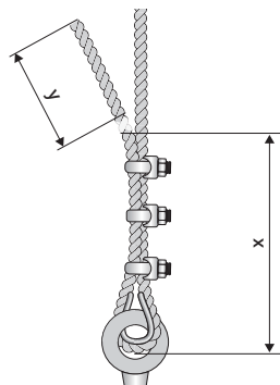
Obr. 30: Náčres zakončení lana pro typ 36, 37
