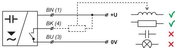
Рис. 11: Подключение датчика с выходом типа NPN (исполнение N, NT)
