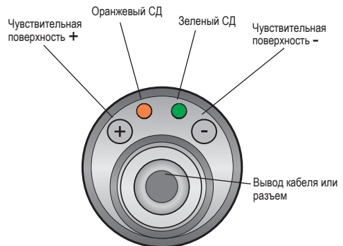
Рис. 15: Вид сверху на датчик
