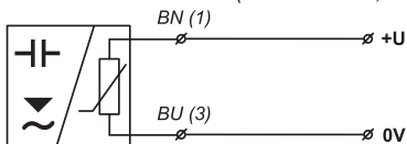
Рис. 13: Подключение датчика с выходом типа NAMUR (исполнение Xi, XiM, XiT, XiMT)
