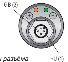
Схема подключения и вид изнутри разъёма уровнемера DLM (вариант - I)
