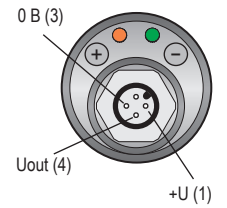
Схема подключения и вид изнутри разъёма уровнемера DLM (вариант - U)
