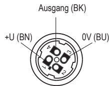
Anordnung der Pins der Steckerdose
