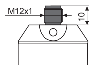
Ausführung „H“ mit Tülle für den Schutzschlauch
