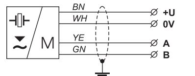
Schaltbild und Innenansicht des Steckers des Füllstandsmessers ULM (Variante - M)
