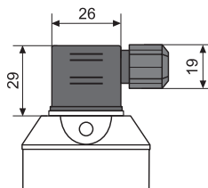
Ausführung „B“ mit kurzer Kabeltülle PG11
