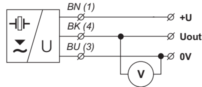
Schaltbild und Innenansicht des Steckers des Füllstandsmessers ULM (Variante - U)
