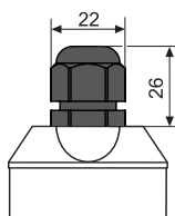
Ausführung „B“ mit kurzer Kabeltülle PG11
