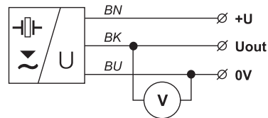
Schaltbild und Innenansicht des Steckers des Füllstandsmessers ULM (Variante - U)
