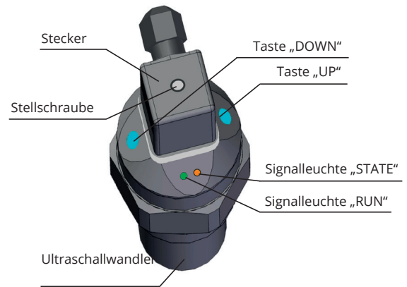
Beschreibung der Hauptbestandteile des Füllstandsmessers - Version mit Tasten
