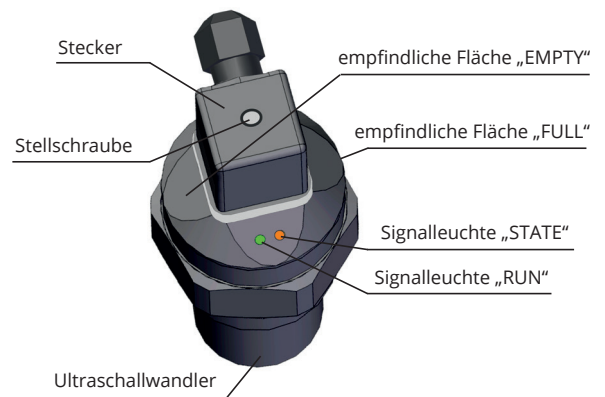
Beschreibung der Hauptbestandteile des Füllstandsmessers mit Halo-Sonden
