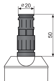
Ausführung „H“ mit Tülle für den Schutzschlauch
