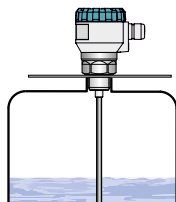
Obr. 8: Instalace hladinoměru v nekovové nádrži
