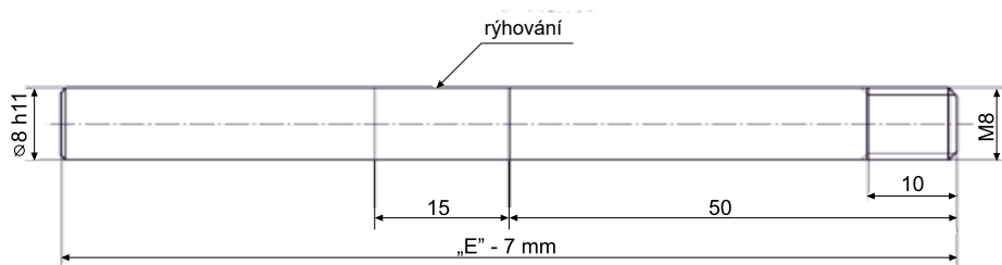
Obr. 25: Detail nákresu tyčové elektrody
