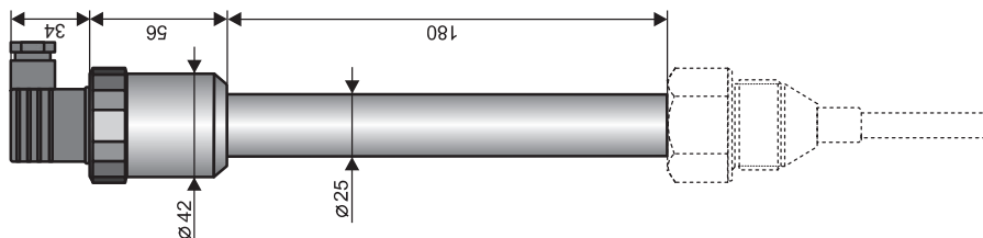
vysokoteplotní provedení CLM-36_T
