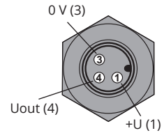
Připojovací schéma a vnitřní pohled na konektor hladinoměru ULM (varianta - I)
