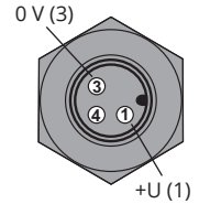
Připojovací schéma a vnitřní pohled na konektor hladinoměru ULM (varianta - I)
