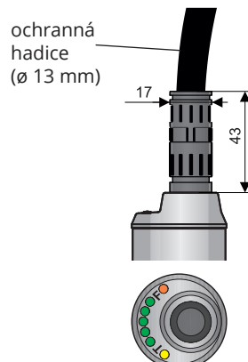
Provedení „H“ s vývodkou pro ochranné hadice - pro použití ve venkovním prostředí nebo v místě zvýšené vlhkosti.
