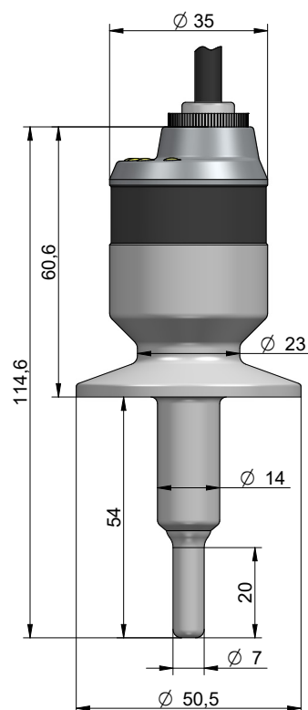
Provedení „C“ s konektorem M12
