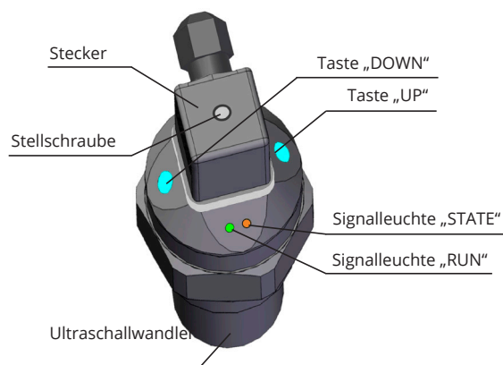
Beschreibung der Hauptbestandteile des Füllstandsmessers - Version mit Tasten
