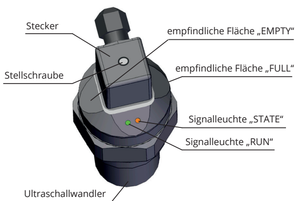
Beschreibung der Hauptbestandteile des Füllstandsmessers mit Hallo-Sonden
