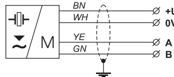
Schaltbild und Innenansicht des Steckers des Füllstandsmessers ULM (Variante - M)
