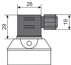
Ausführung „B“ mit kurzer Kabeltülle PG11
