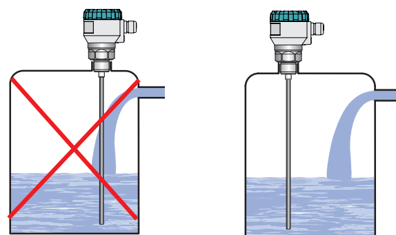
Рис. 11: Установка уровнемера вне доступа потока наполнения
